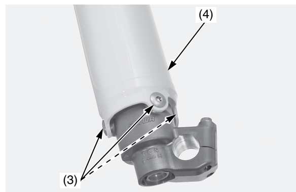
(3) bulloni a brugola dell'elemento di protezione della forcella (4) elemento di protezione della forcella
