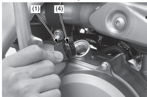
(1) tappo di rifornimento dell'olio del cambio (4) O-ring
