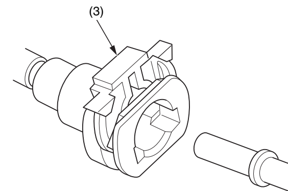
(3) fermo scorrevole
