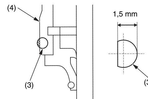
(3) anelli di usura (4) tubo esterno
