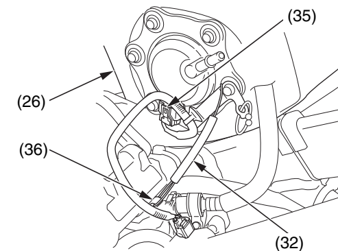
(26) serbatoio del carburante (35) connettore della pompa del carburante B (32) cavo del fermo (36) gancio sul telaio
