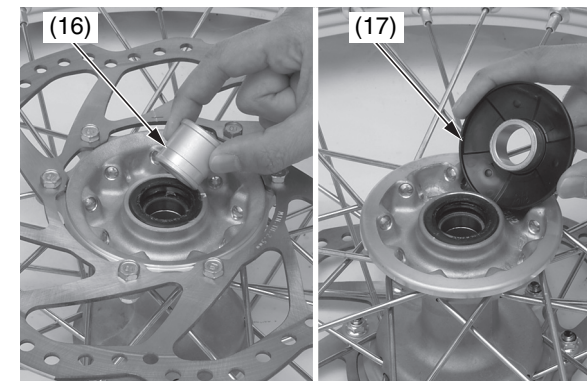
(16) collare sinistro (17) collare destro
