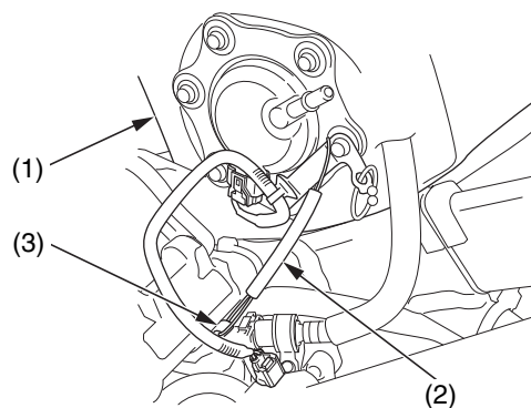
(1) serbatoio del carburante (2) cavo del fermo (3) gancio sul telaio
