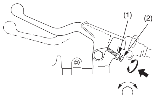
(1) dado di bloccaggio (2) registro
