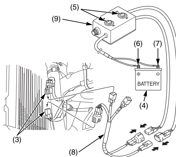
(3) connettori del cablaggio secondario del DLC/pompa del carburante (4) batteria da 12 V (5) selettori del cablaggio della batteria (6) cavo positivo (+) del cablaggio della batteria (7) cavo negativo (-) del cablaggio della batteria (8) adattatore del cablaggio della batteria (9) cablaggio della batteria
