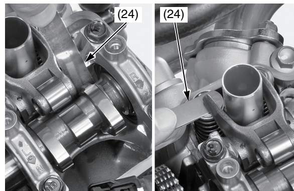
(24) spessore
