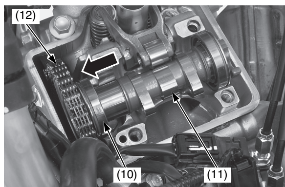
(10) cuscinetto sinistro dell'albero a camme (11) albero a camme (12) catena della distribuzione
