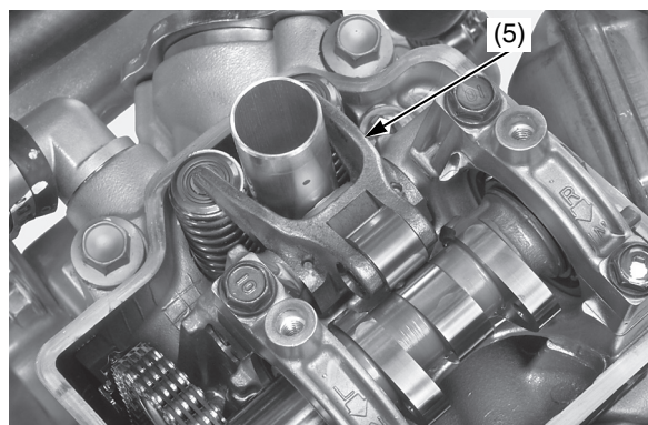
(5) bilanciante di scarico
