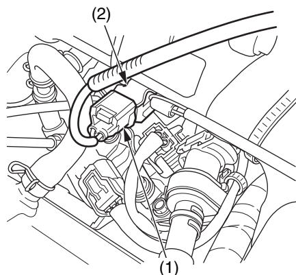
(1) connettore della pompa del carburante A (2) supporto carburante
