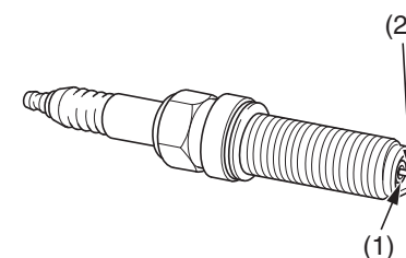
(1) isolatore di porcellana (2) elettrodo centrale
