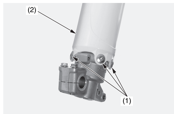
(1) bulloni a brugola dell'elemento di protezione della forcella (2) elemento di protezione della forcella
