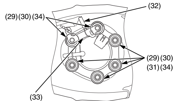
(29) rondelle elastiche coniche (30) collari (31) rondelle (32) cavo del fermo (33) guida del cavo del fermo (34) bulloni di fissaggio della pompa del carburante
