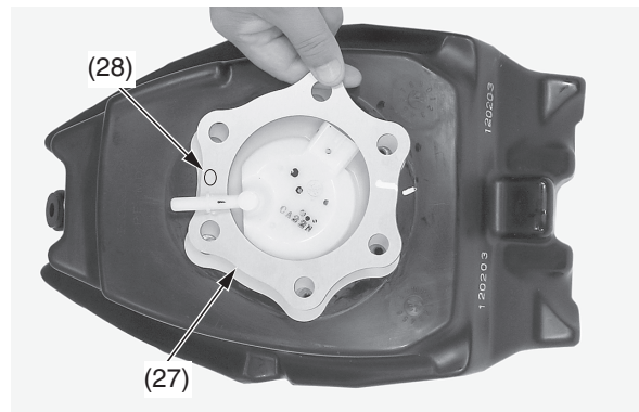
(27) piastra della pompa del carburante (28) segno identificativo
