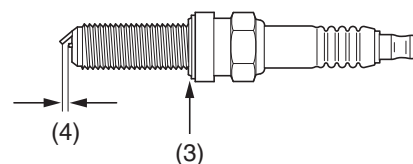
(3) guarnizione di tenuta (4) distanza tra gli elettrodi della candela
