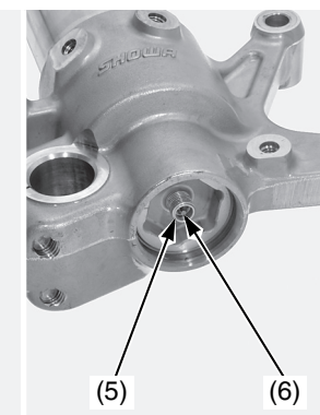
(3) valvola dell'aria della camera interna (4) valvola dell'aria della camera esterna (5) valvola dell'aria della camera di bilanciamento (6) elemento centrale della valvola dell'aria della camera di bilanciamento
