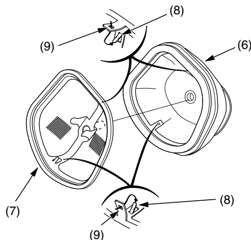
(6) filtro aria (7) portafiltro (8) linguette del portafiltro (9) fori
