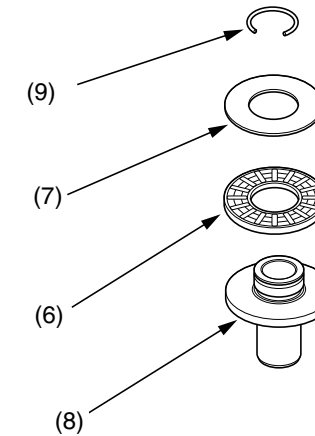
(6) cuscinetto ad aghi (7) rondella
