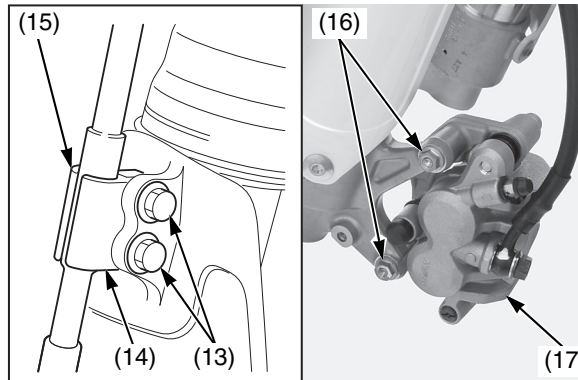
(13) bulloni del morsetto del tubo flessibile del freno (14) supporto A (15) supporto B (16) bulloni di fissaggio della pinza del freno anteriore (17) pinza del freno
