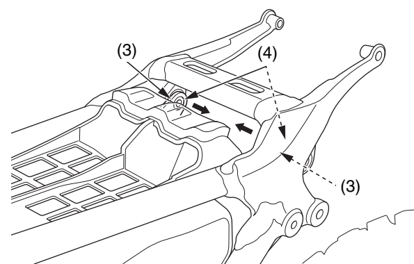
(3) scatola del filtro dell'aria (4) borchie telaio secondario
