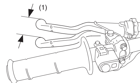
(1) gioco
