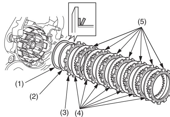
(1) sede della molla (2) molla antivibrations (3) disco conduttore A della frizione
