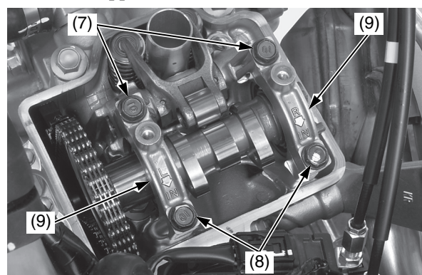
(7) bulloni del supporto dell'albero a camme A (8) bulloni del supporto dell'albero a camme B (9) anelli di posizionamento e supporti dell'albero a camme
