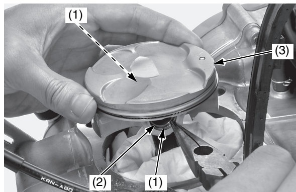
(1) fermagli dello spinotto del pistone (3) pistone (2) spinotto del pistone
