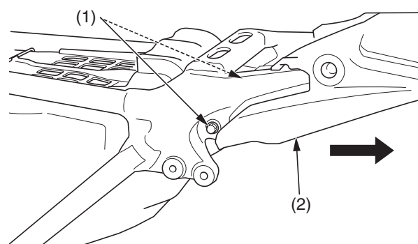
(1) bulloni e dadi di fissaggio del parafango posteriore (2) parafango posteriore
