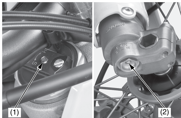
(1) vite di regolazione dello smorzamento della compressione (2) vite del registro di smorzamento dell'estensione
