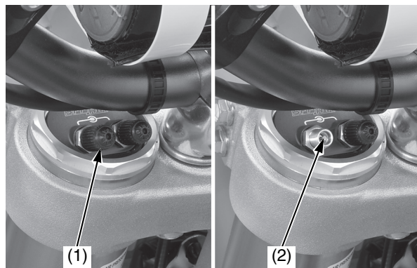
(1) tappo della valvola (2) valvola dell'aria della camera interna
