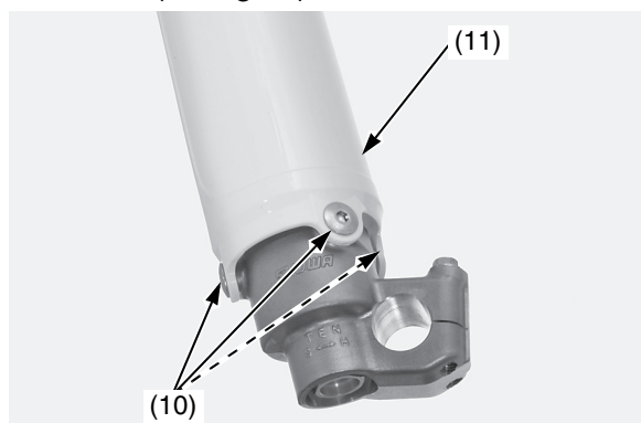
(10) bulloni a brugola dell'elemento di protezione della forcella (11) elemento di protezione della forcella
