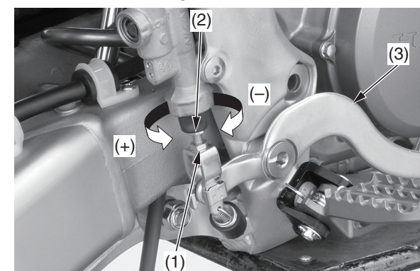
(1) dado di bloccaggio (2) puntale (3) pedale del freno posteriore (+) sollevamento del pedale del freno (-) abbassamento del pedale del freno
