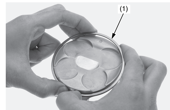
(1) fascia elastica
