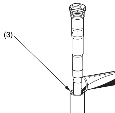
(3) tubo esterno
