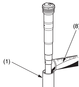
(1) gruppo della forcella (8) olio della forcella
