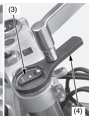
(4) chiave inglese
