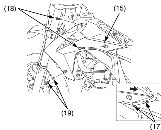
(15) protezioni (17) linguette del coperchio dell'alloggiamento del filtro dell'aria (18) bulloni B della protezione (19) collari e bulloni A della protezione
