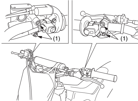
(1) bulloni di fissaggio delle leve dei comandi
