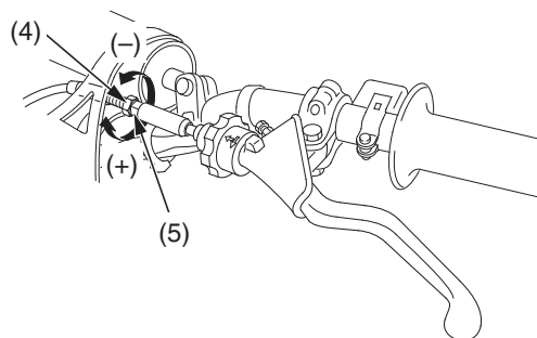
(4) dado di bloccaggio (5) registro incorporato nel cavo (+) aumento del gioco (-) diminuzione del gioco
