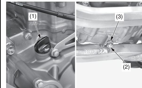
(1) tappo di rifornimento/astina di livello dell'olio motore (2) vite di scarico dell'olio motore (3) rondella di tenuta (nuova)
