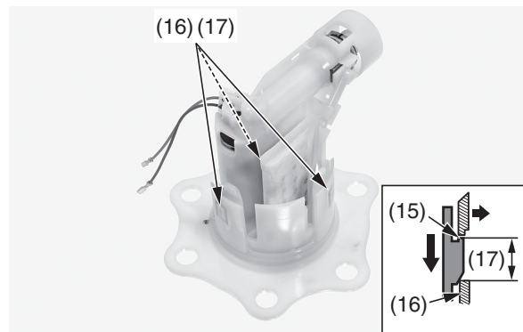
(15) ganci (16) linguette
