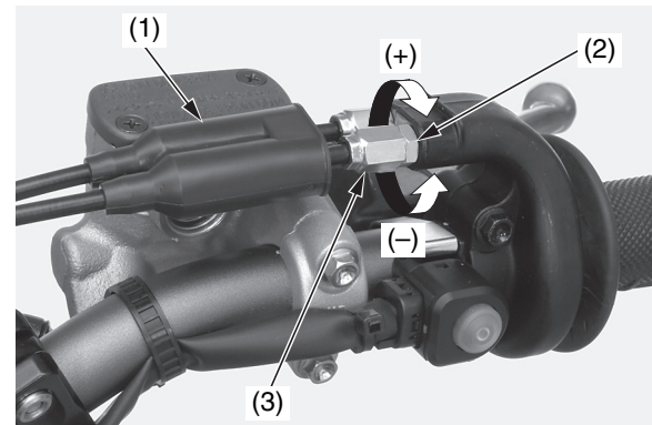
(1) parapolvere (+) aumento del gioco (2) dado di bloccaggio (–) diminuzione del gioco (3) registro
