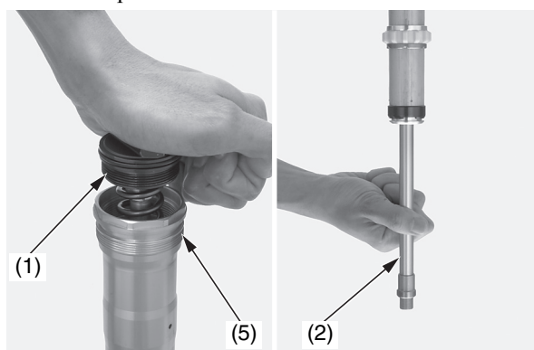
(1) tappo della forcella (2) asta dell'ammortizzatore forcella (5) ammortizzatore della forcella
