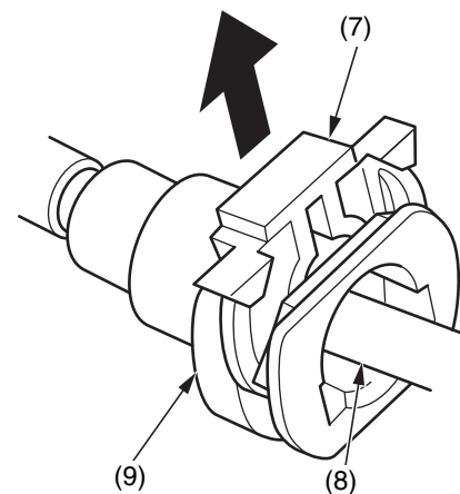
(7) fermo scorrevole (8) giunto del carburante (9) alloggiamento del connettore
