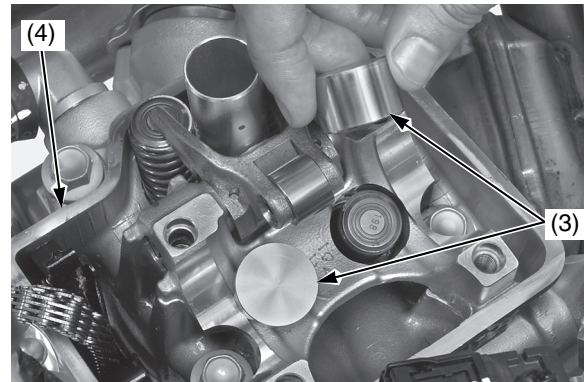
(3) alzavalvole (4) testata
