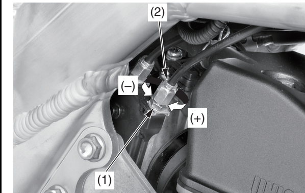
(1) dado di bloccaggio (+) aumento del gioco (2) registro (–) diminuzione del gioco
