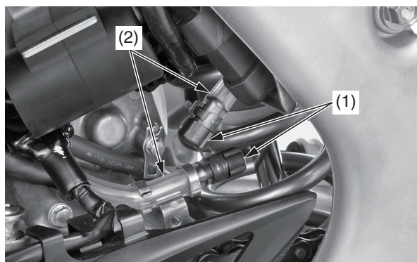
(1) tappi dei tubi di sfiato del basamento (2) tubi di sfiato del basamento
