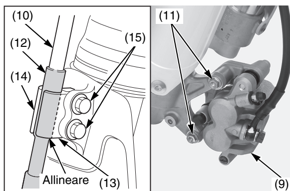
(9) pinza del freno (10) tubo flessibile del freno (11) bulloni di fissaggio della pinza del freno anteriore (12) protezione tubo flessibile del freno (13) supporto A (14) supporto B (15) bulloni del morsetto del tubo flessibile del freno
