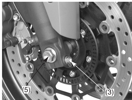
(5) Bullone dell'assale
