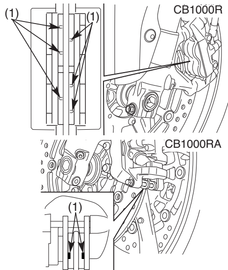
(1) Segno di indicazione usura
