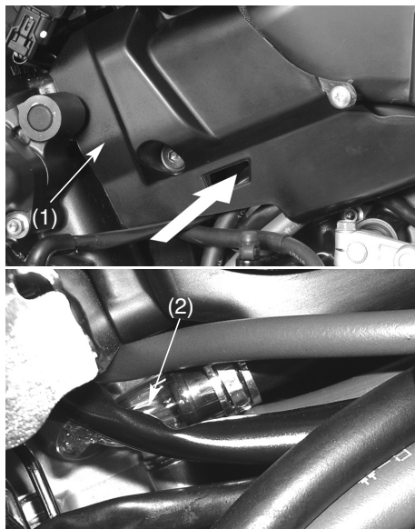
(1) Coperchio
