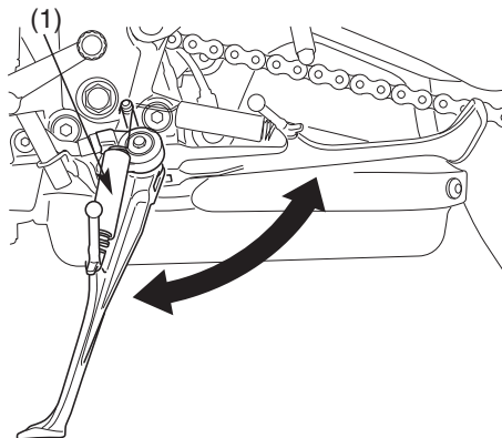
(1) Molla del cavalletto
