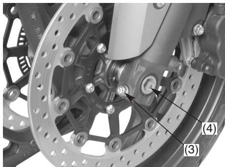
(3) Bulloni serraggio dell'assale (4) Assale anteriore
