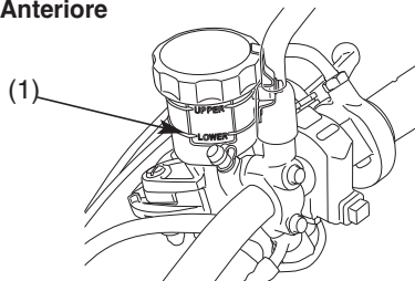
(1) Contrassegno del livello inferiore (LOWER)
