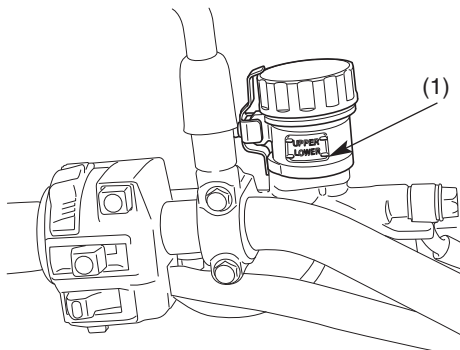
(1) Contrassegno del livello inferiore (LOWER)
