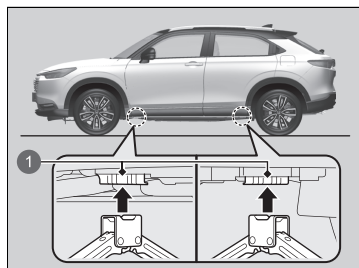
1 Punti di sollevamento
