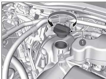
❶ Tappo di riempimento olio motore
