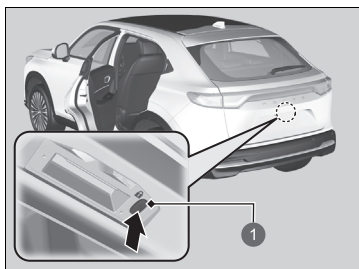
1 Pulsante di blocco portiere
