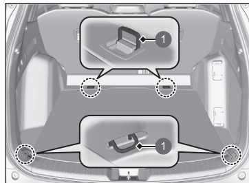
1 Ancoraggi
