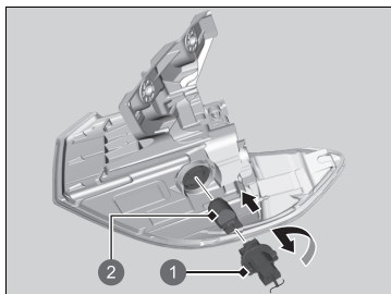
1 Portalampada 2 Lampadina
