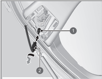
1 Lampadina 2 Portalampada
